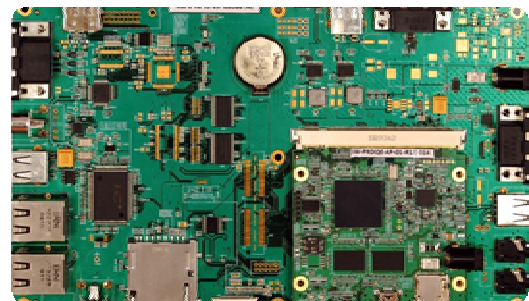
i.MX51 SOM用キャリアボード (写真はSOM搭載済み)
